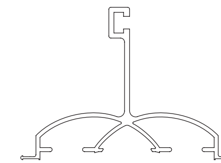
Sezione del montante Upright cross section
